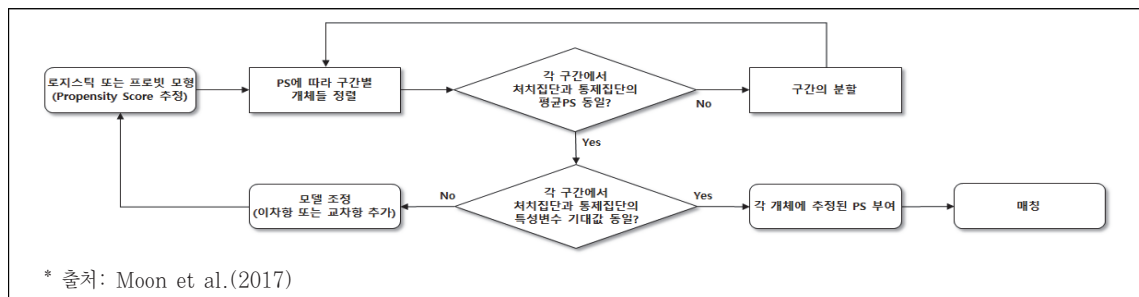
〈Figure 1〉 PS추정 알고리즘
