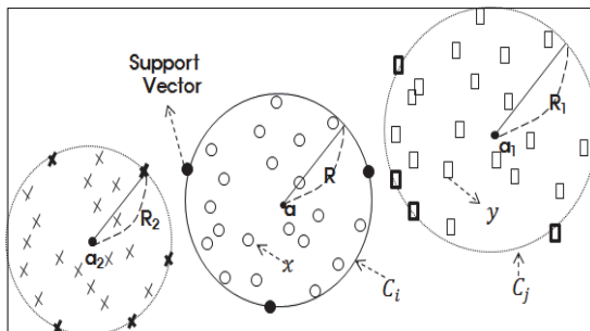
〈그림 2〉 SVDD를 반영한 군집화
